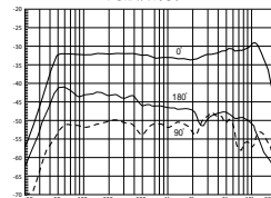
SGM-3416L 周波数特性
