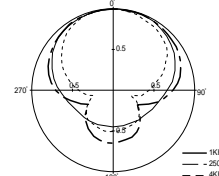
指向特性
