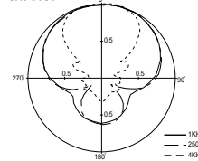
指向特性
