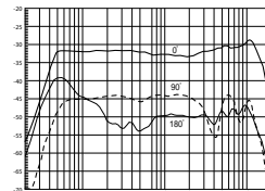
SGM-3416 周波数特性
